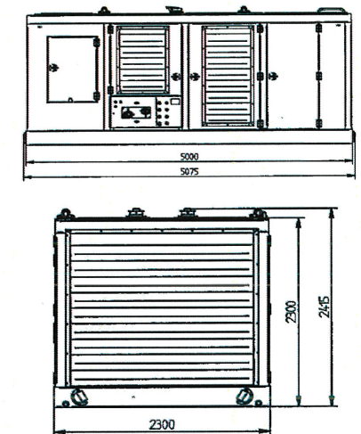
【 2.パワーパック図面 】
