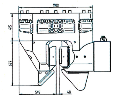
【 3.シングルチャック図面 】
